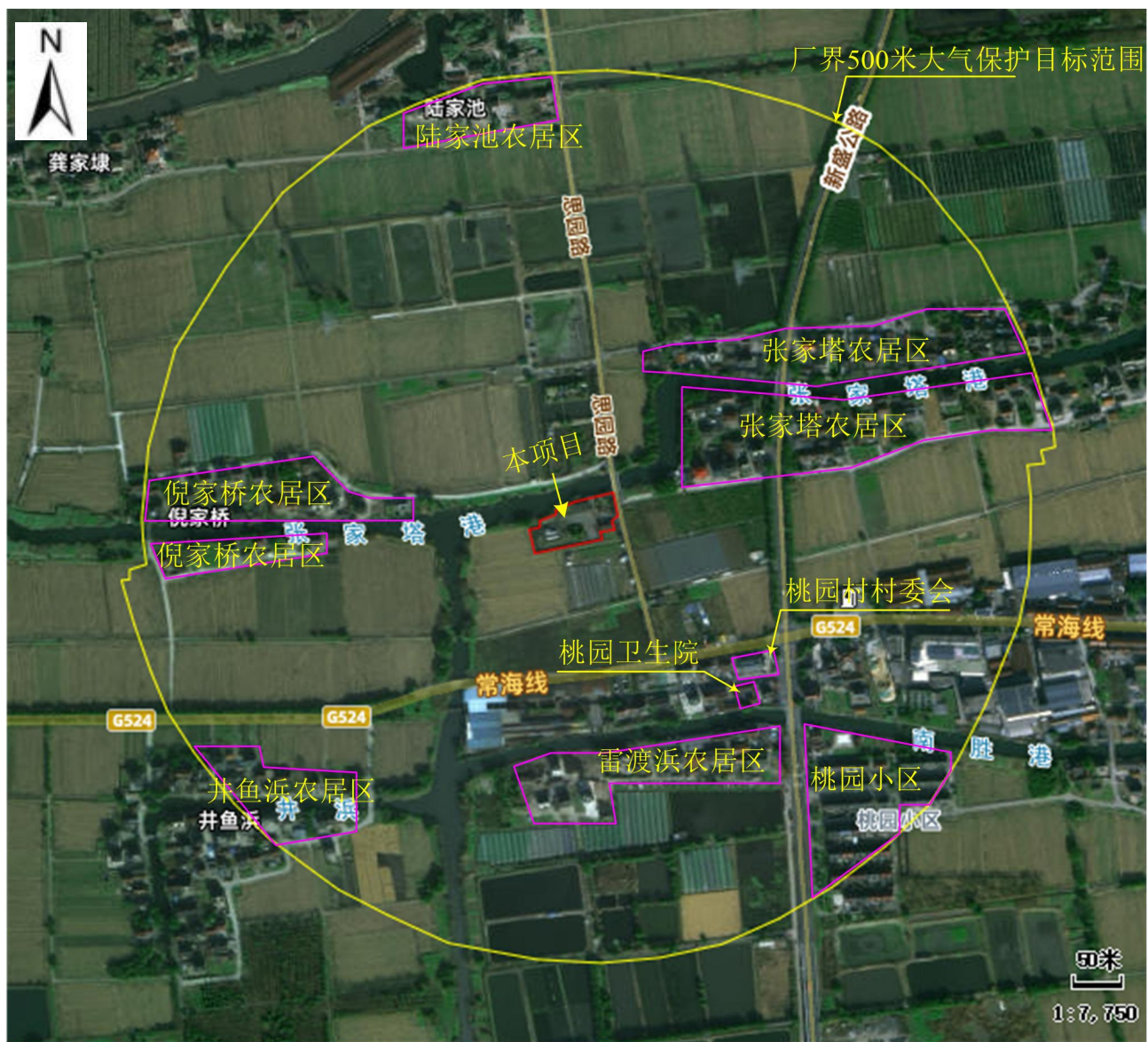
附图 7 建设项目周围近距离环境示意图
