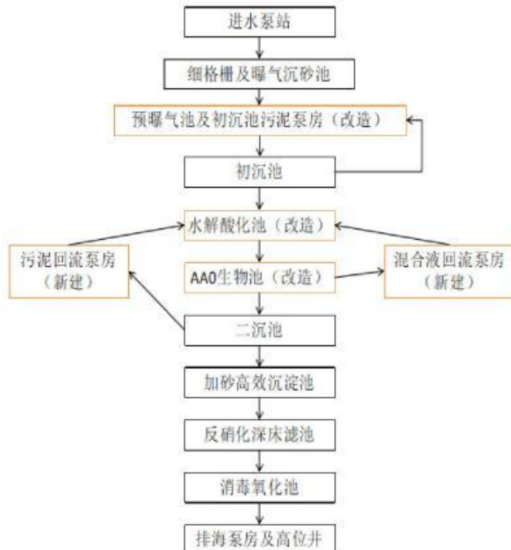
图 4-2 清洁排放提标改造后污水处理厂二期工程工艺流程图
