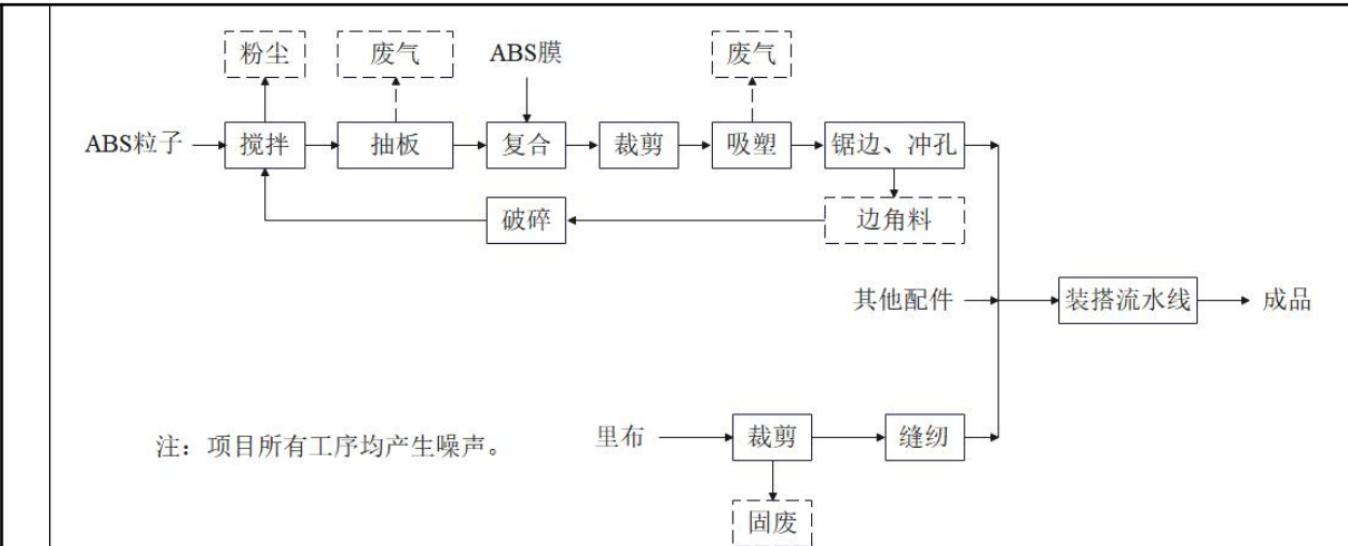
图 2-3 项目箱包生产工艺流程及产污环节示意图
